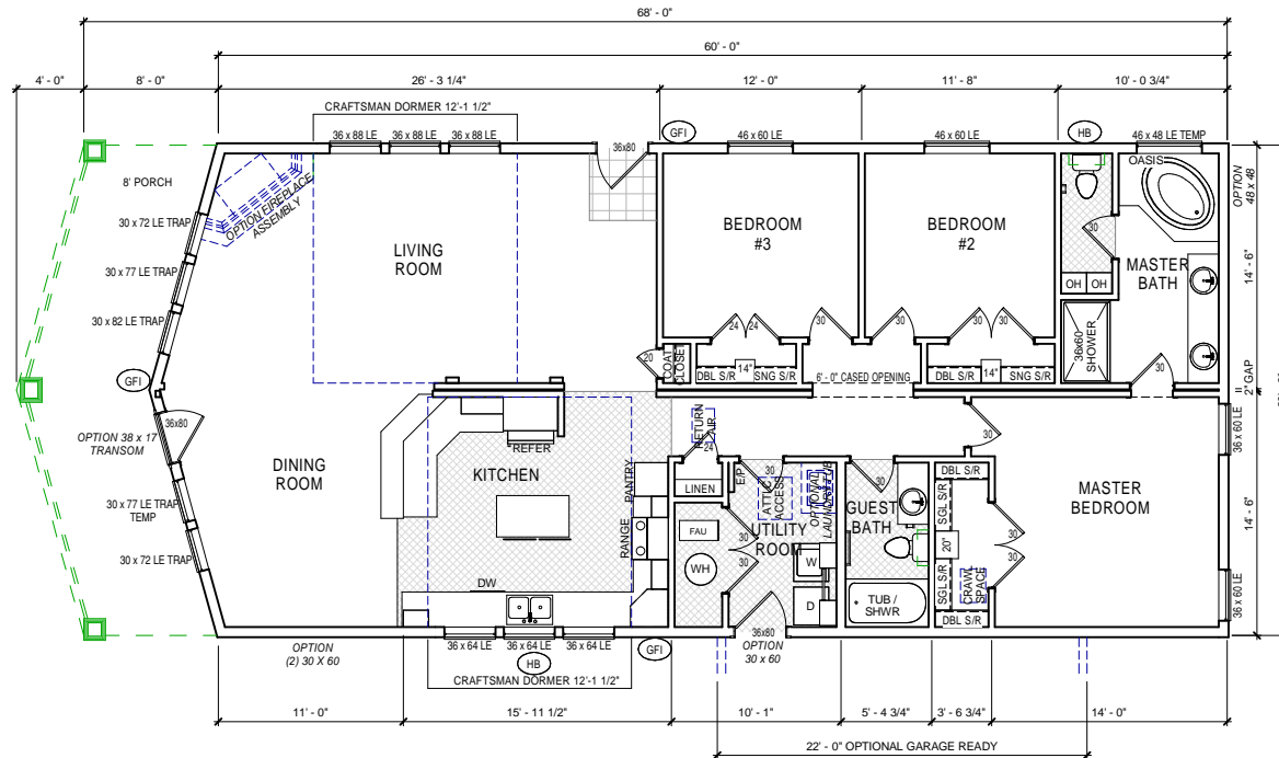
L1-Sales Floor Plan N.T.S.
