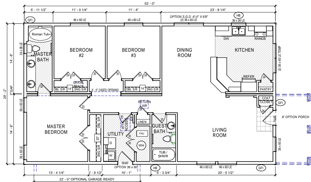
L1-Sales Floor Plan N.T.S.
